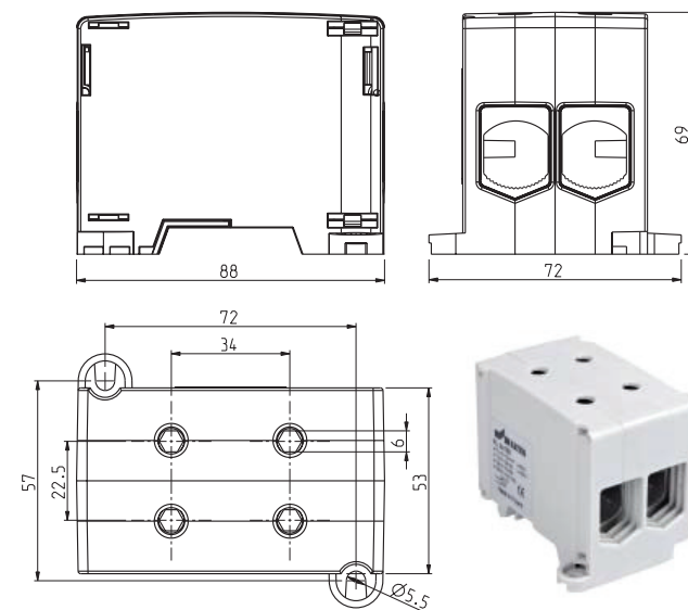
KL 2X150
