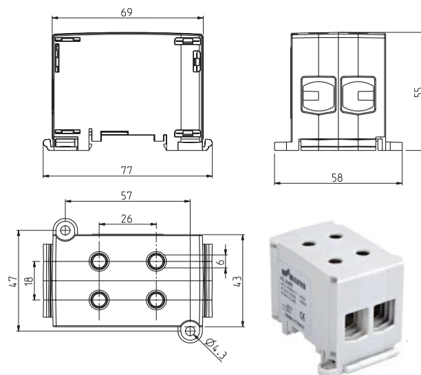
KL 2X95
