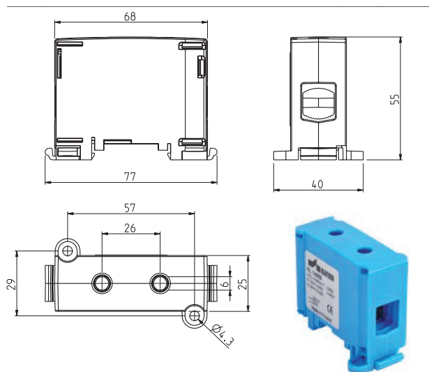
KL 1X95
