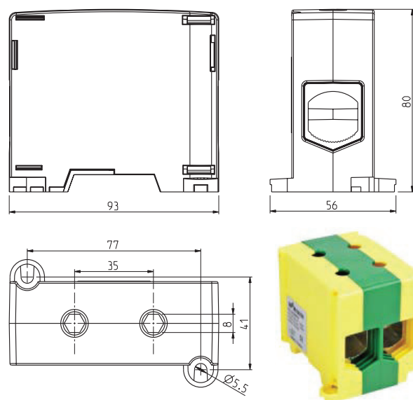
KL 2X240
